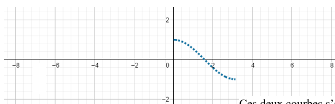
Courbe représentative de la fonction \cos
